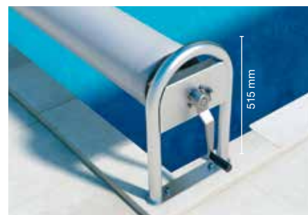
Aufrollvorrichtung «balu» Enroulement modèle «balu»
